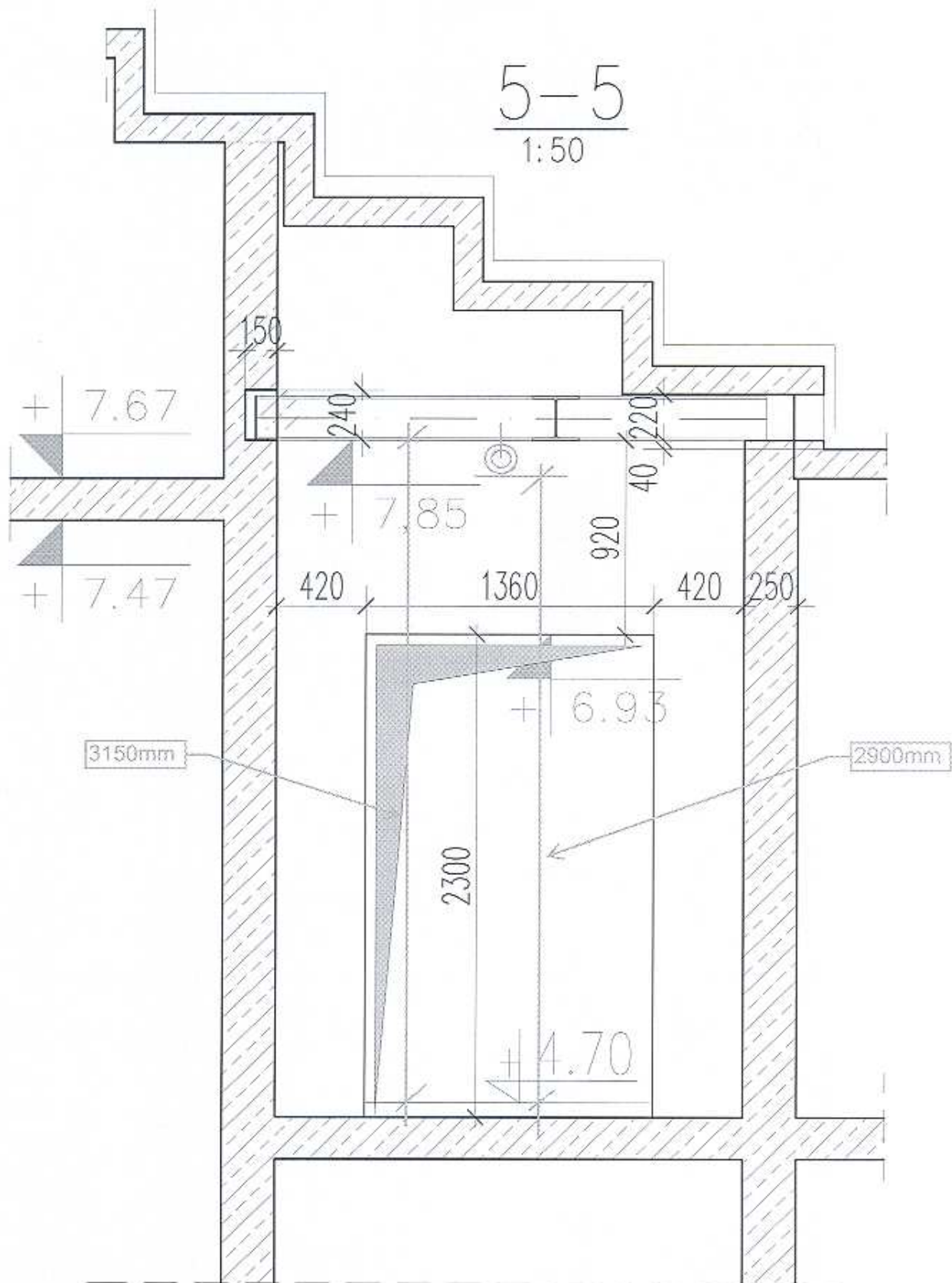
Nadszybie W-02
